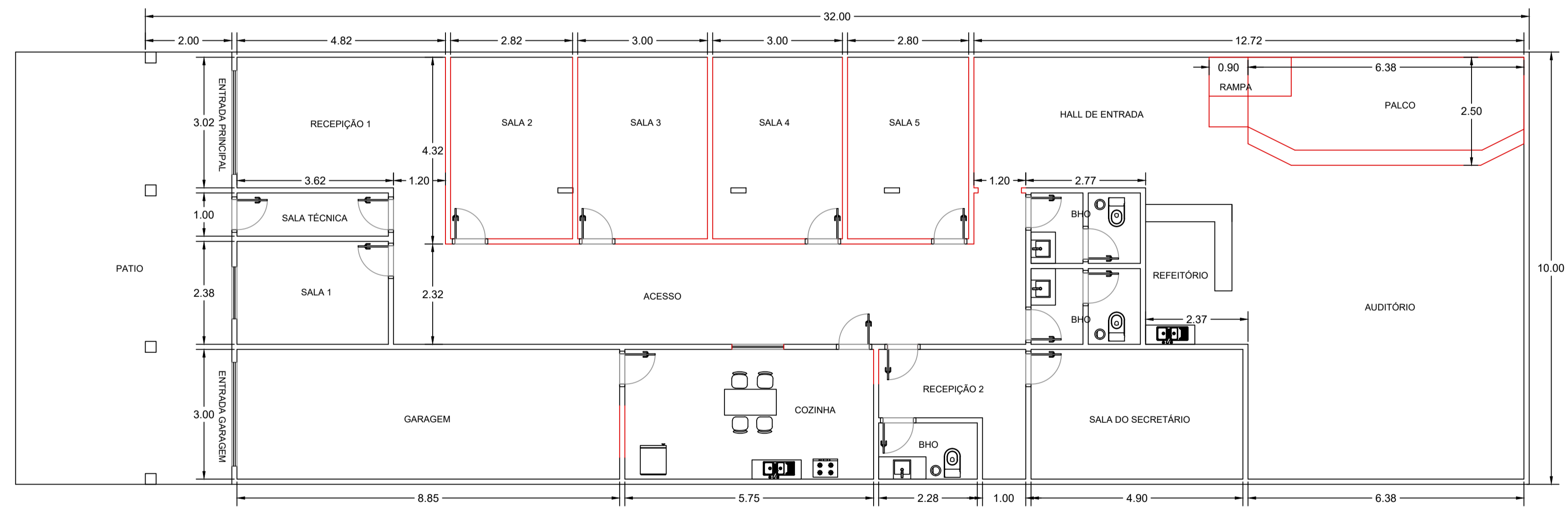
PLANTA BAIXA (COM REFORMA) escala 1:175
